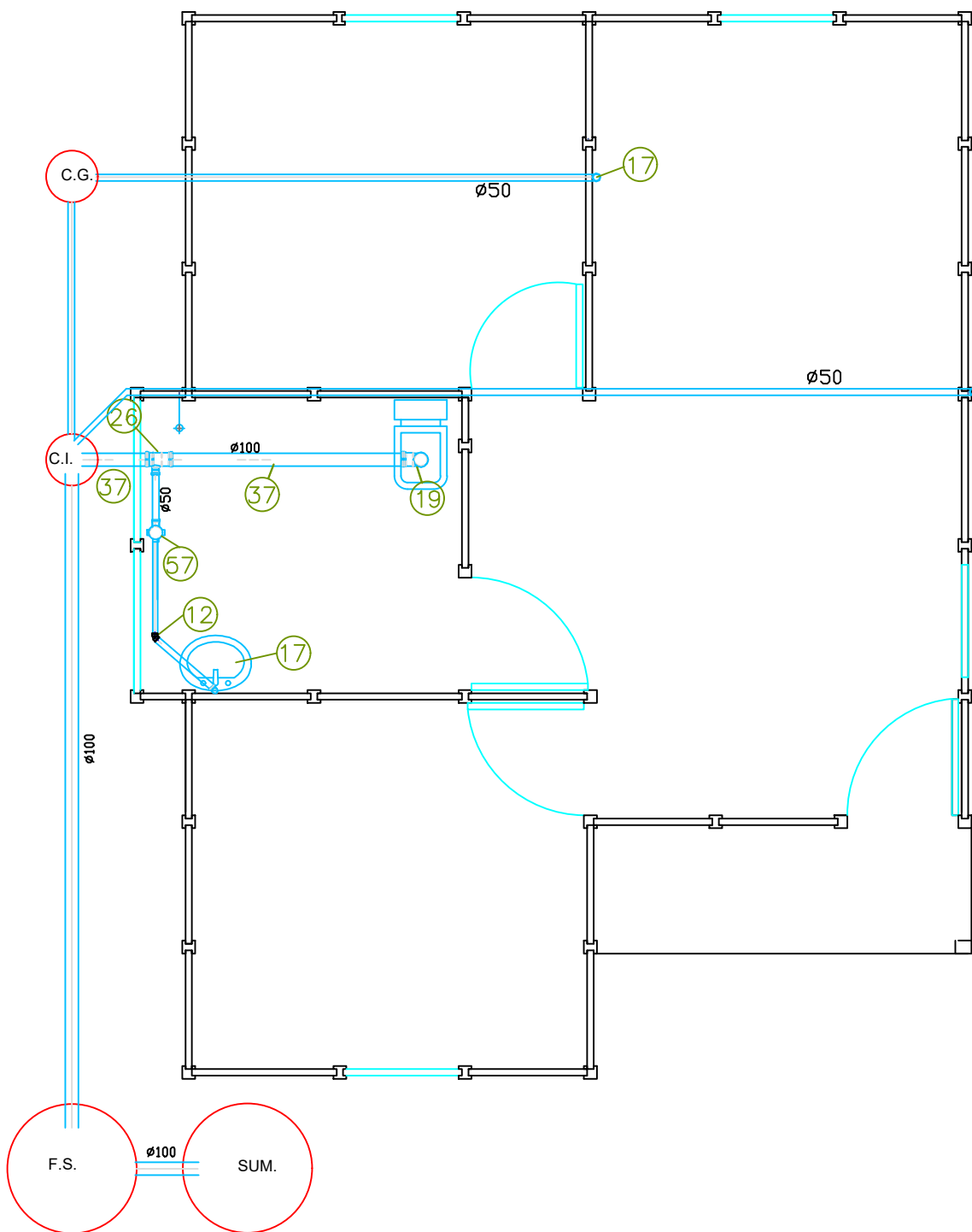
DISTRIBUIÇÃO ÁGUA FRIA ESCALA:.....1/50
