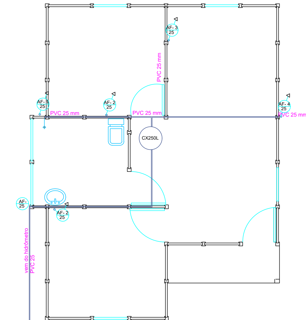
DISTRIBUIÇÃO ÁGUA FRIA ESCALA:.....1/50
