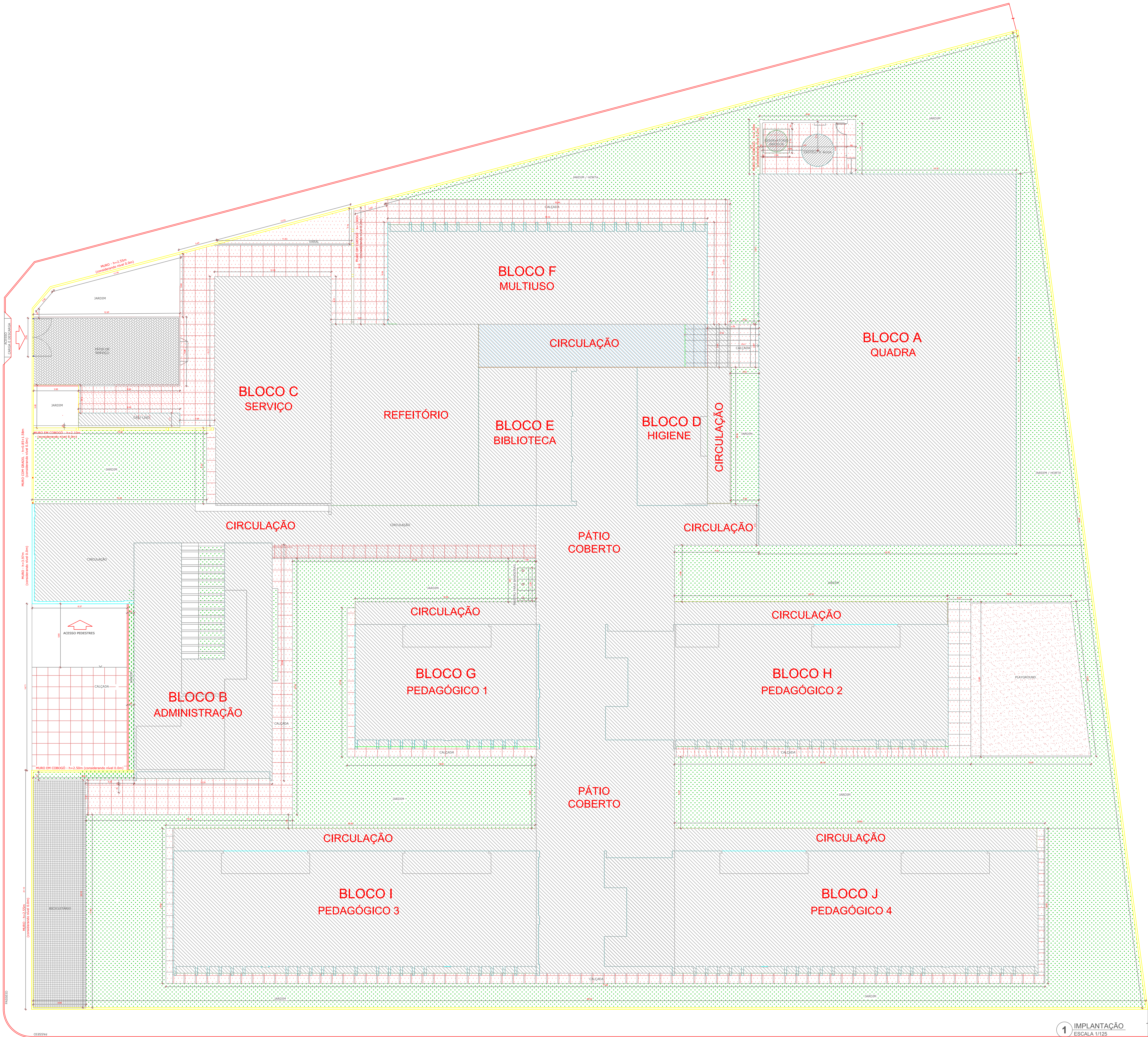
1 IMPLANTAÇÃO ESCALA 1/125
