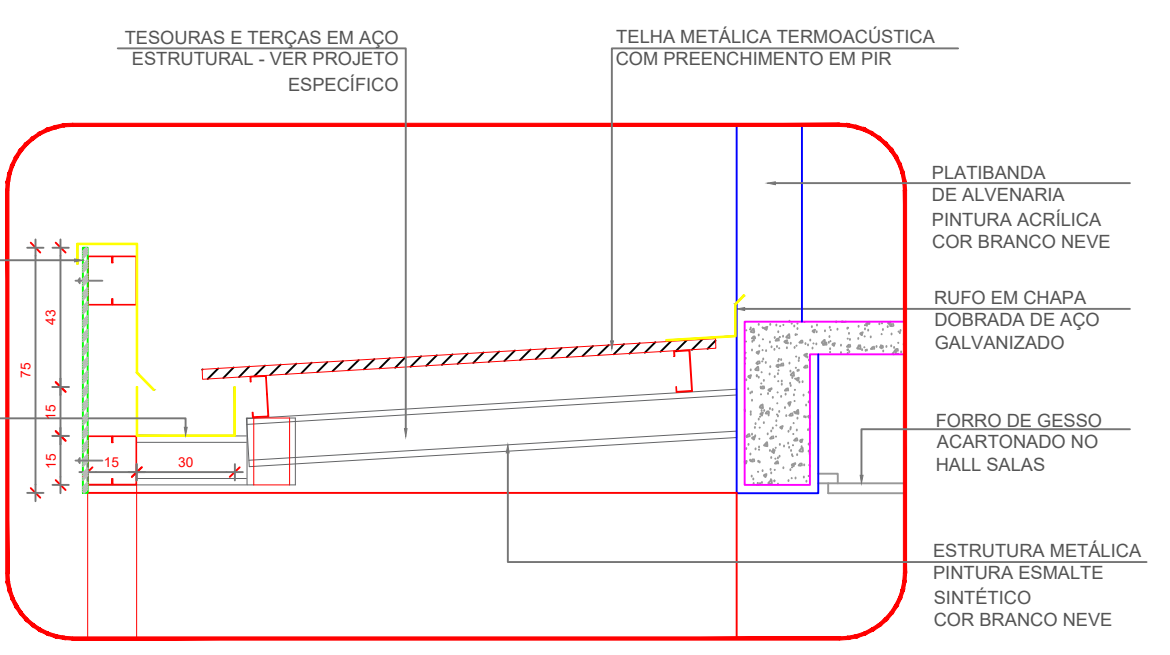
6 DETALHE 2 - PASSARELAS ESCALA 1/20
