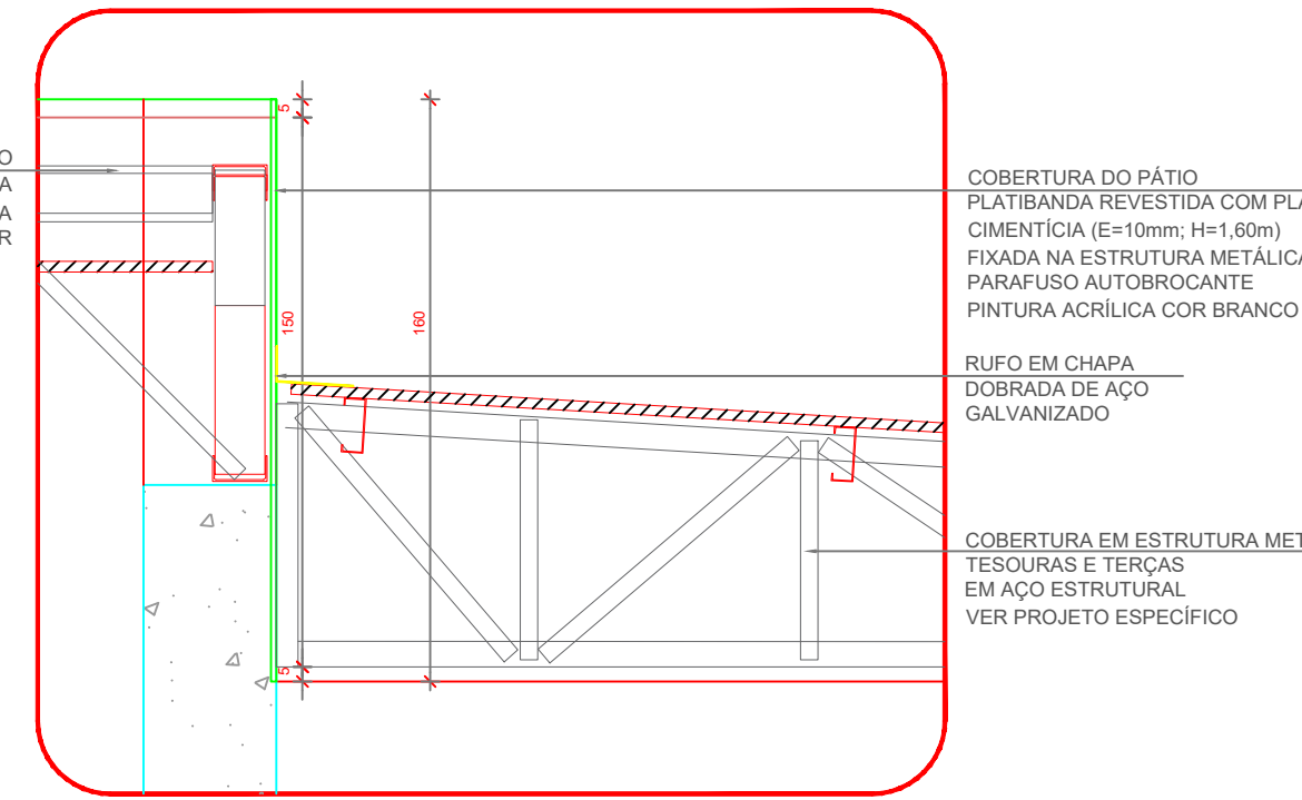
7 DETALHE 3 - PÁTIO COBERTO ESCALA 1/25
