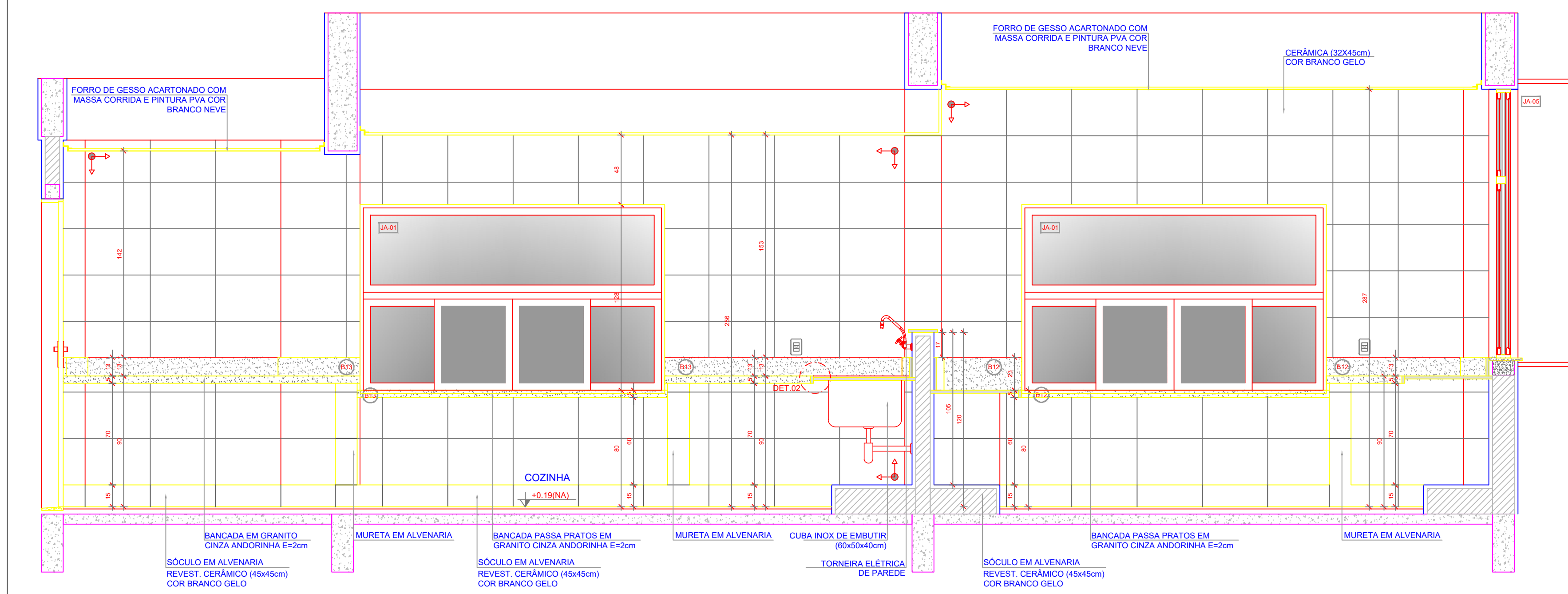
DETALHE 1 - CORTE bancada de granito - área seca sem escala
