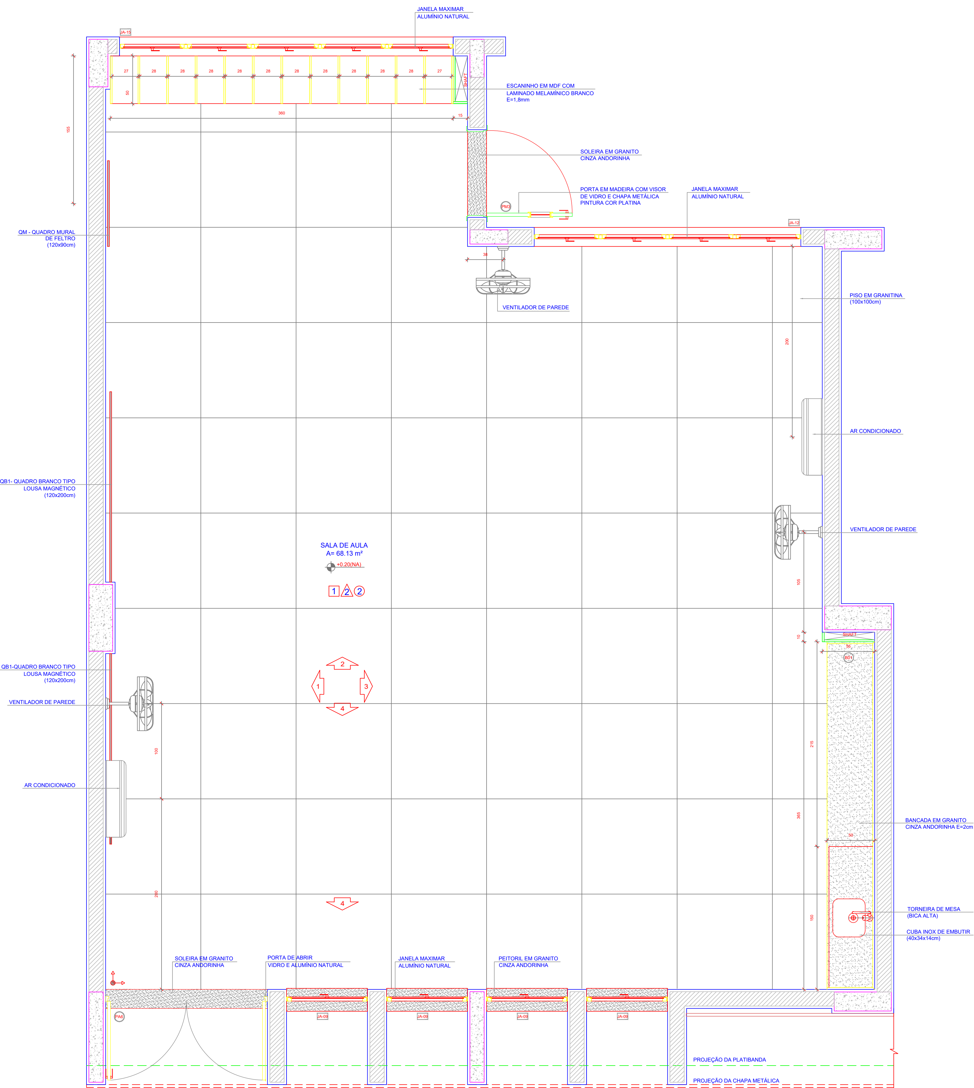
PLANTA BAIXA
