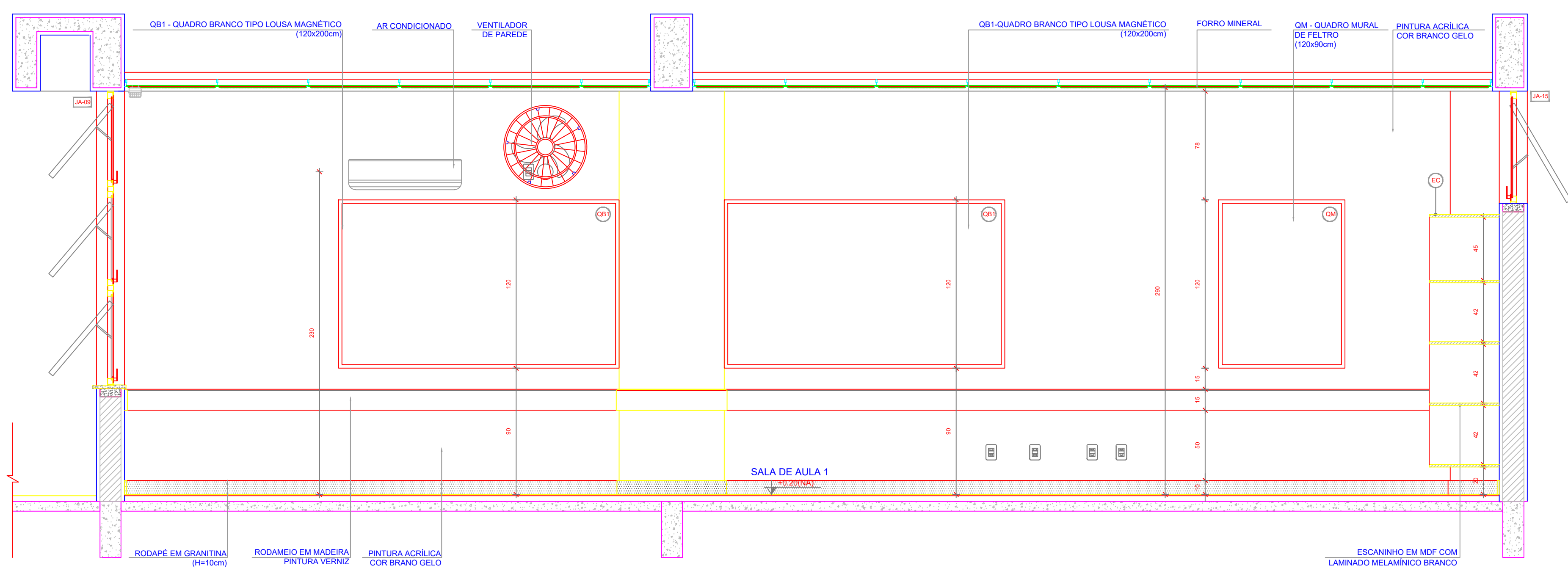
VISTA 1
