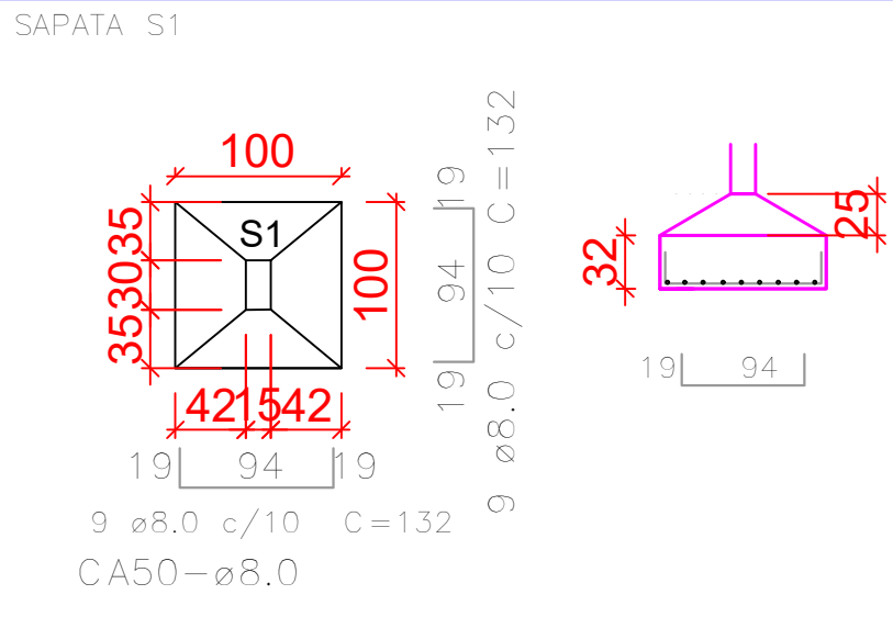
ESTRUTURAS (SAPATA E ESTACAS FACHADA)
