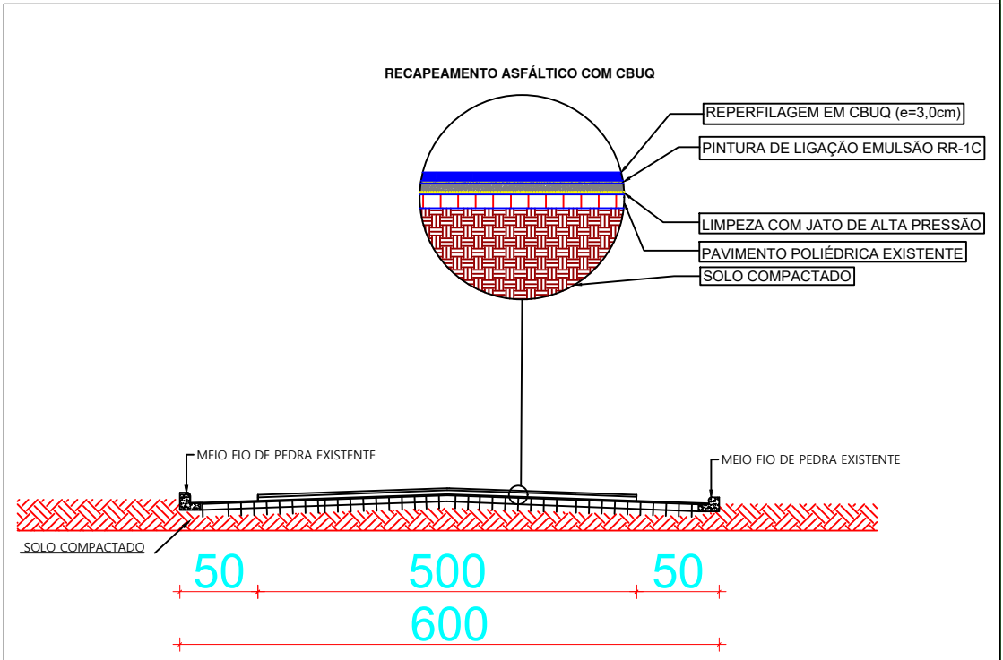
PERFIL TRANSVERSAL DAS VIAS CALÇAMENTADAS SEM ESCALA
