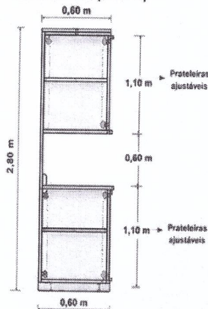
CORTE LATERAL (INTERNO)
