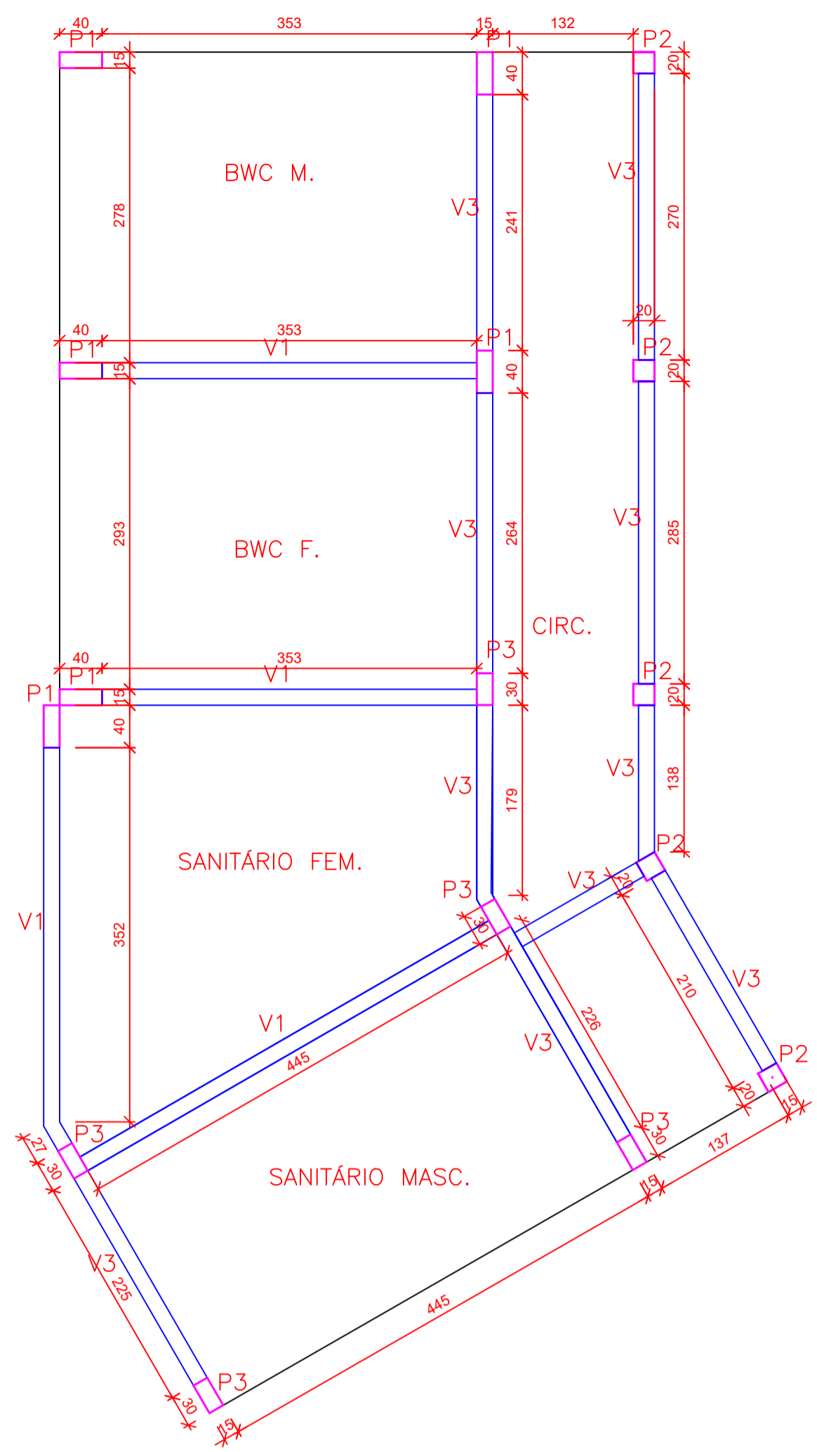
PLANTA BALDRAME - BANHEIROS ESCALA 1:50
