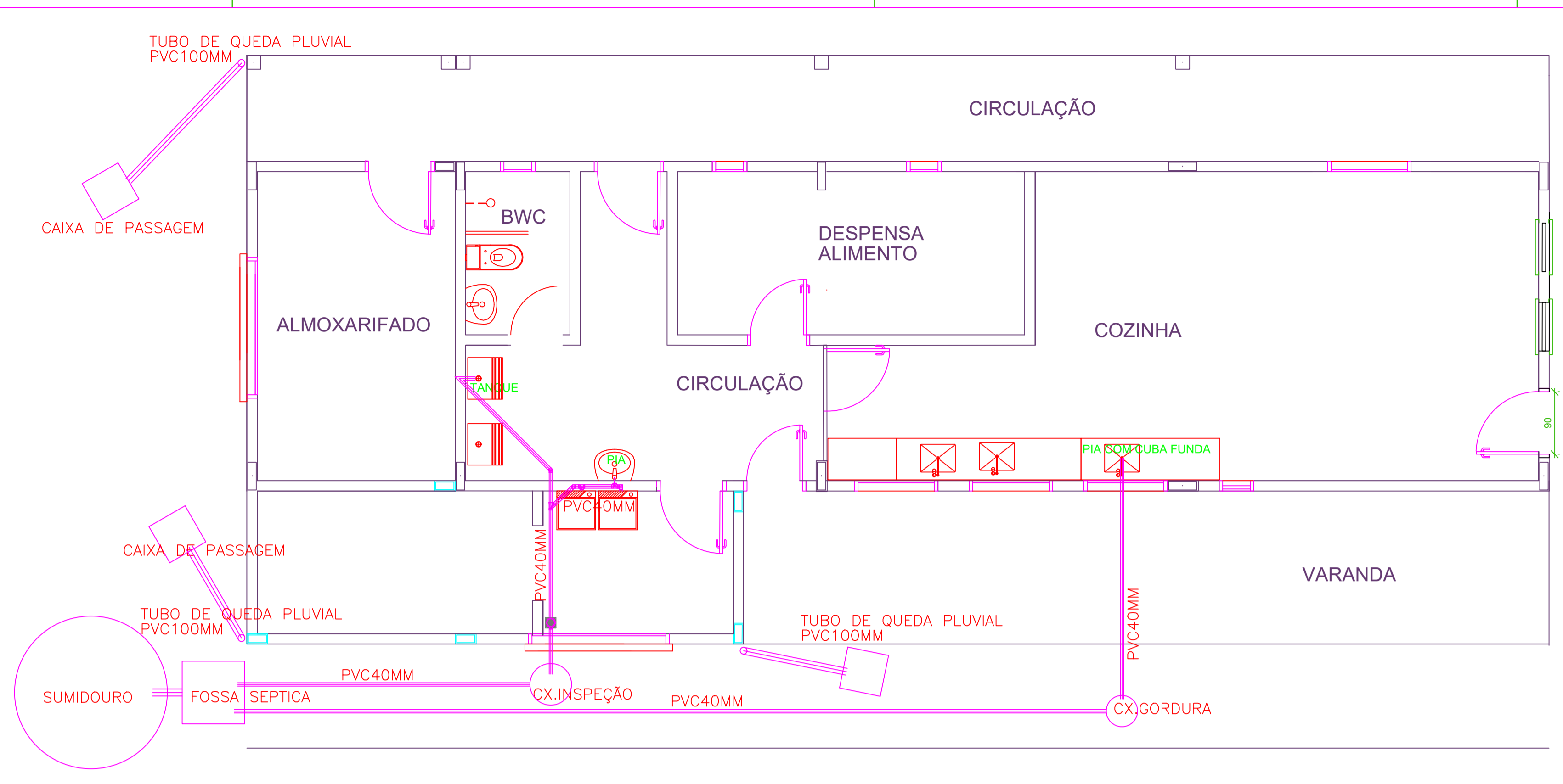
PLANTA BAIXA - COZINHA ESCALA 1/50
