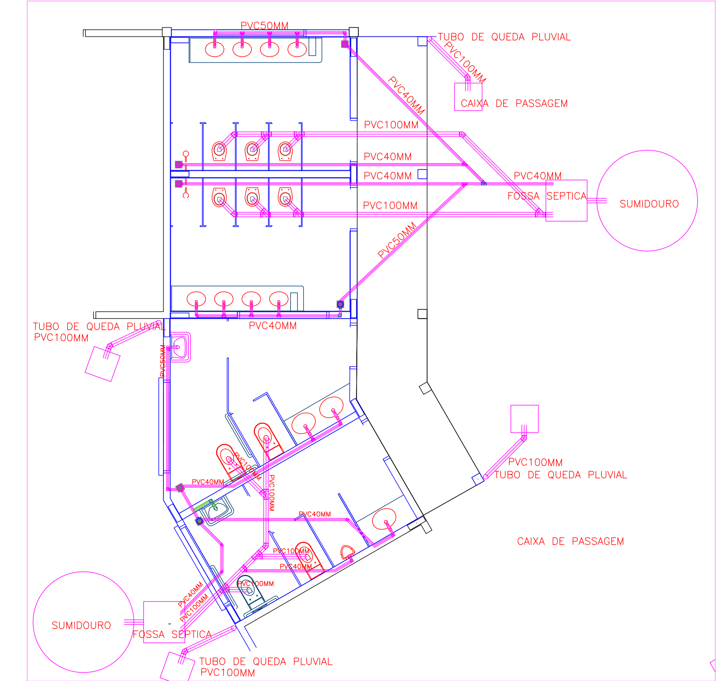
PLANTA SANITÁRIO - BANHEIROS ESCALA 1/50
