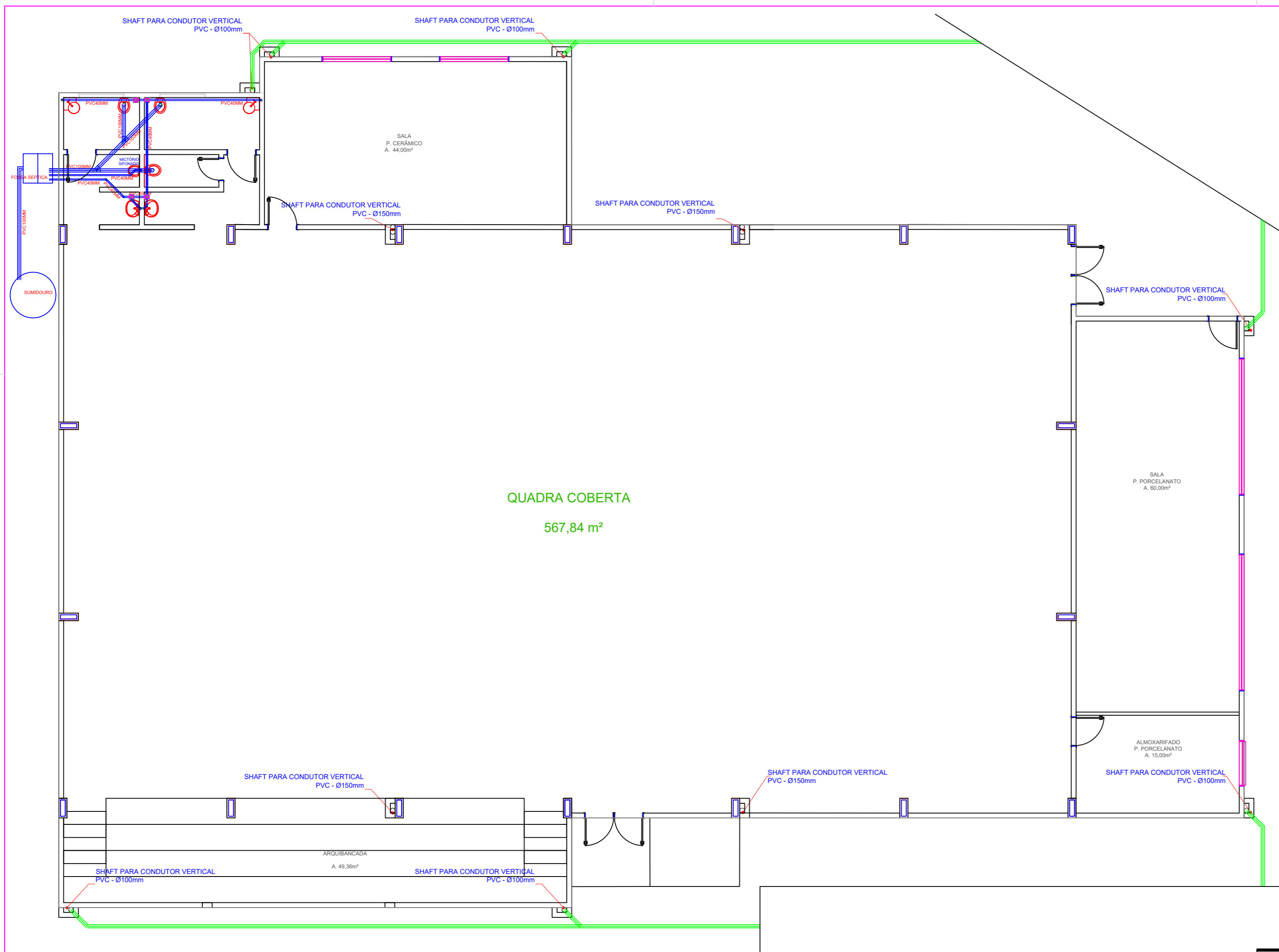
PLANTA BAIXA - SANITÁRIO/PLUVIAL ESCALA 1/50
