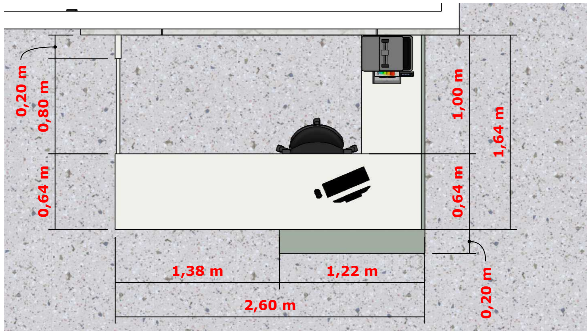
PLANTA BAIXA ESC 1/20
