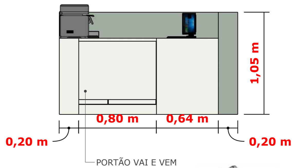
ELEVAÇÃO ESQUERDA ESC 1/20MM
