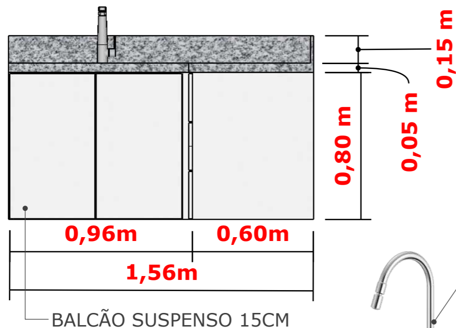
ELEVAÇÃO A ESC 1/20mm
