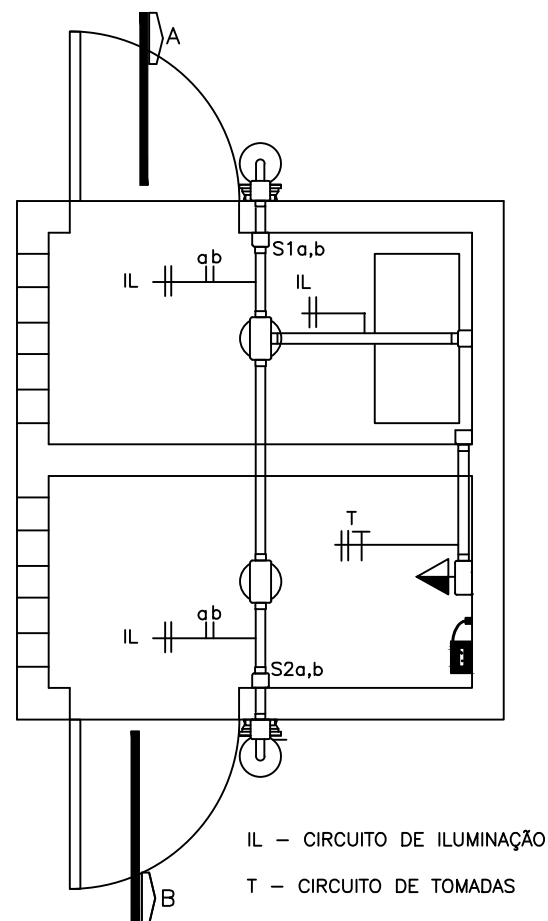
PLANTA BAIXA SEM ESCALA
