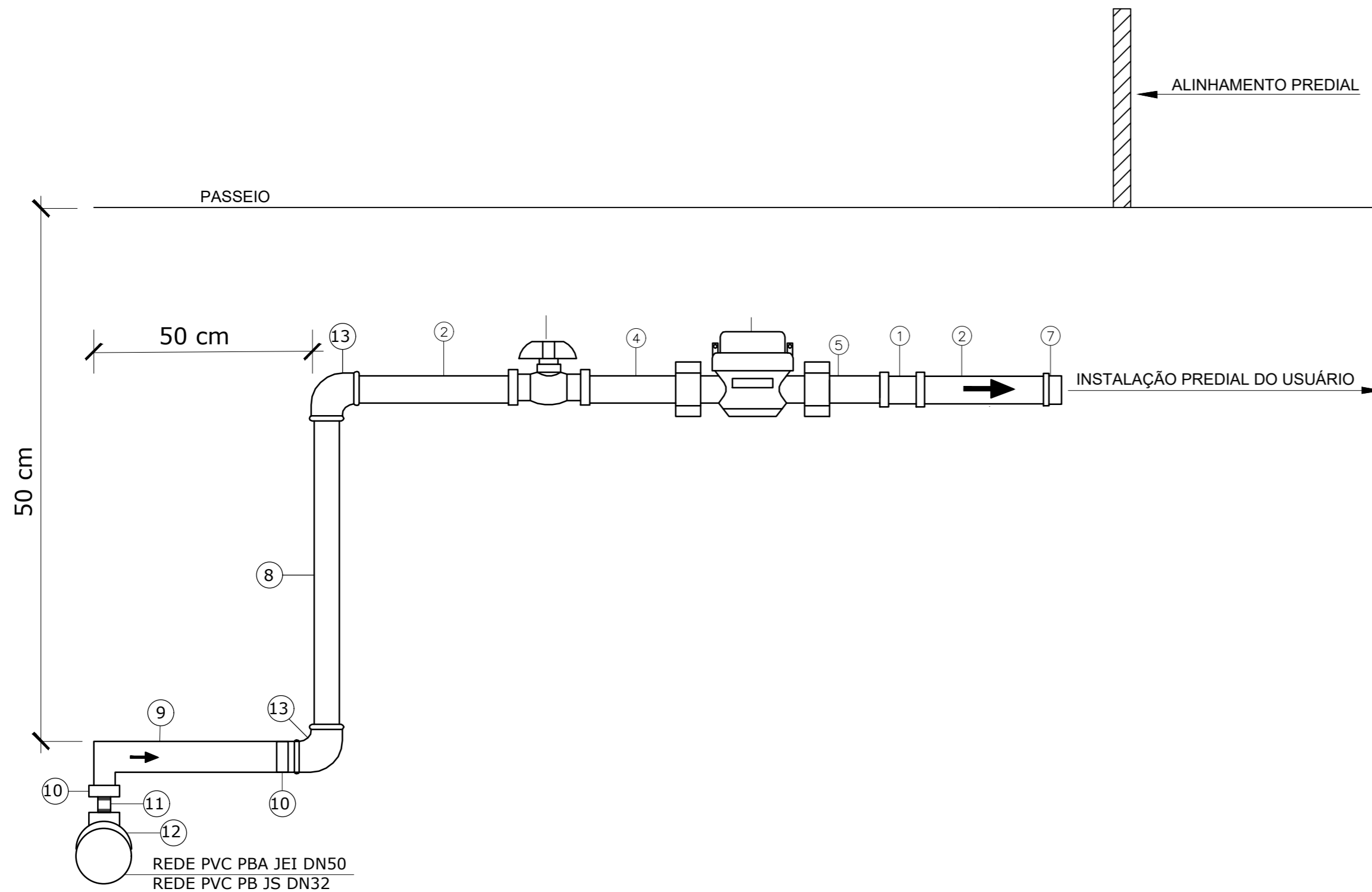
DETALHE DA LIGAÇÃO - HIDRÔMETRO Ø 3/4" Sem escala
