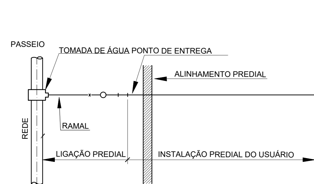
PLANTA BAIXA DA LIGAÇÃO Sem escala
